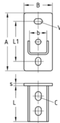
MPC-Sattelflansch, längs
